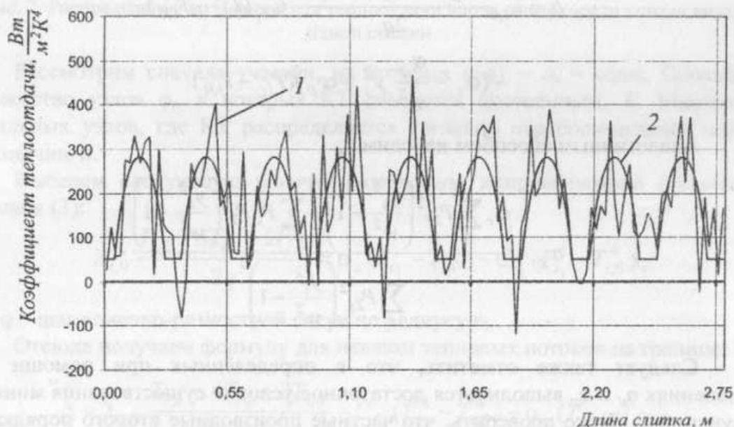
Рис. 3. Результаты определения коэффициента теплоотдачи: 1 – методом прямого обращения; 2 – методом наименьших квадратов
