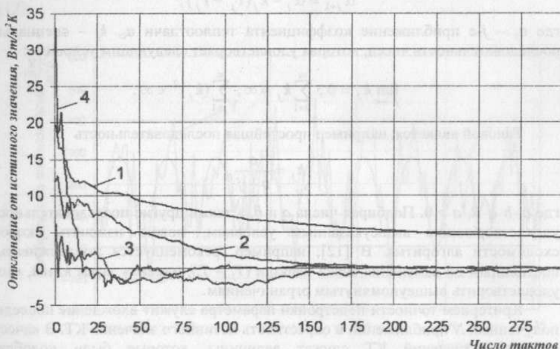
Рис. 4. Траектории подстройки параметров, характеризующие отклонение подстраиваемого параметра от истинного значения.
